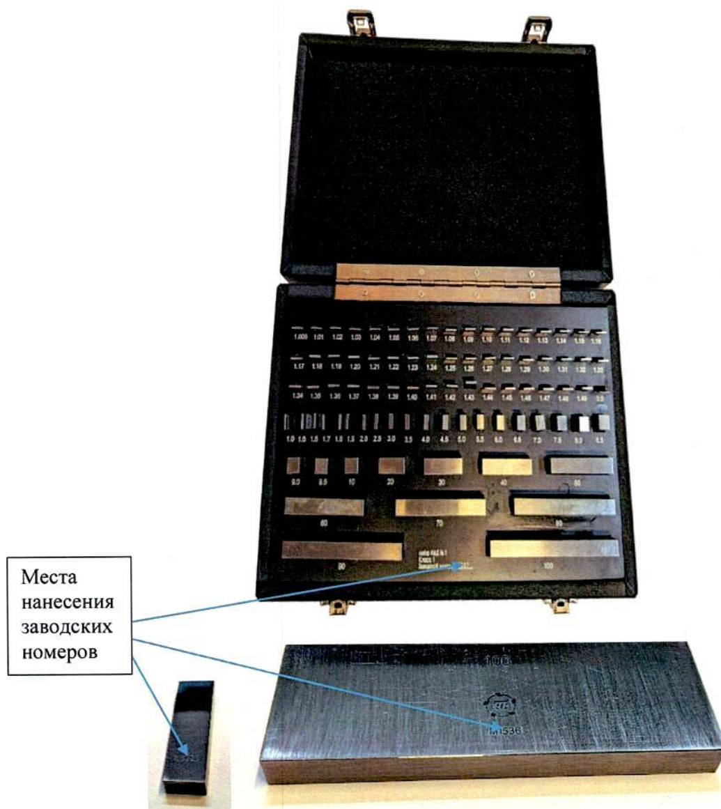
Рисунок 1 – Общий вид концевых мер (лист 1 из 2)
